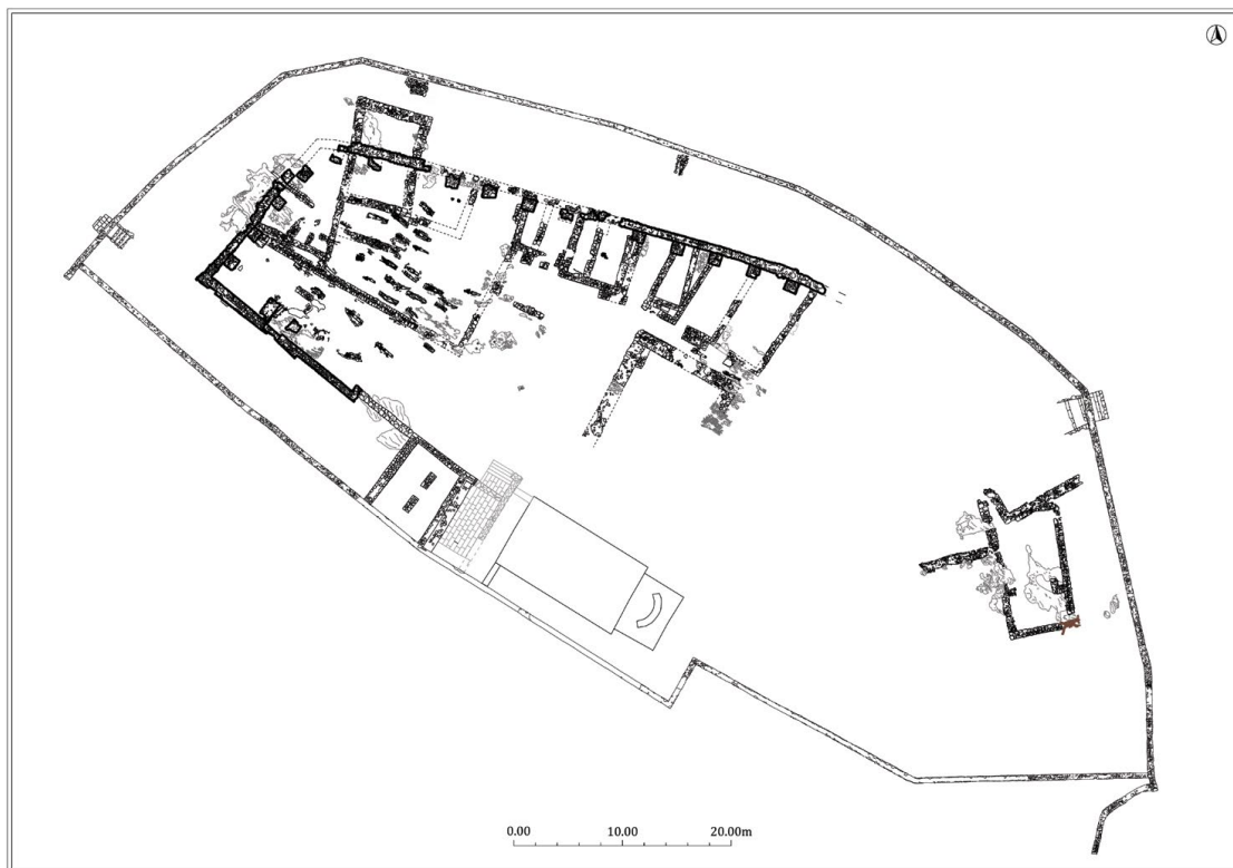
Karta 1 Tlocrtni izgled kasnoantičke utvrde na Sv. Petru u Makarskoj s vanjskim ogradnim zidom iz 17. st. (crtež: Marin Kraljev – Arheorad d.o.o.)
